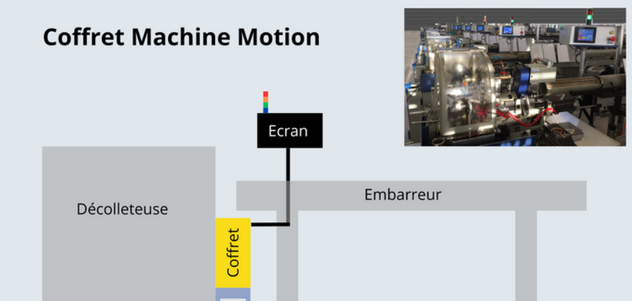
Schéma de l'installation
